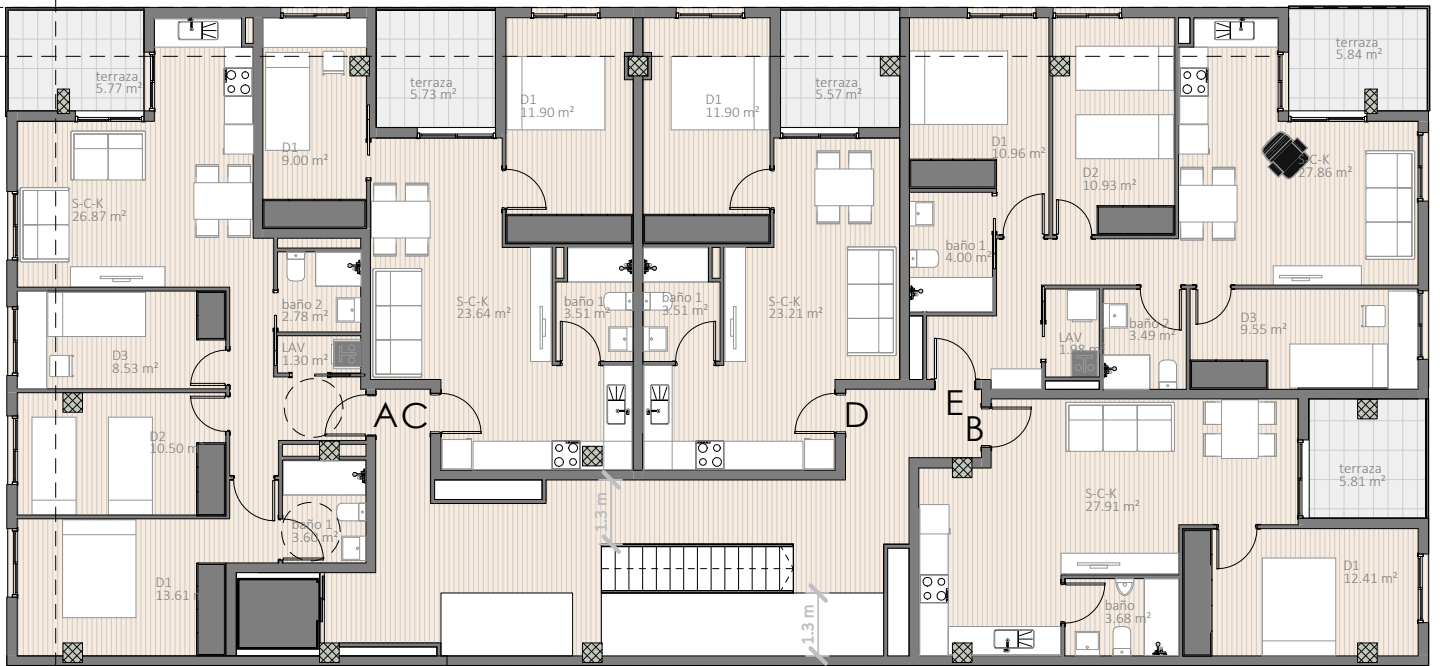
PLANTA TIPO - P1/P2/P3
