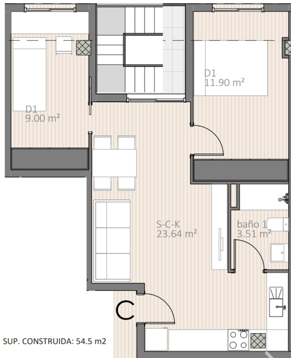
PLANTA CUARTA – VIVIENDA 4C
